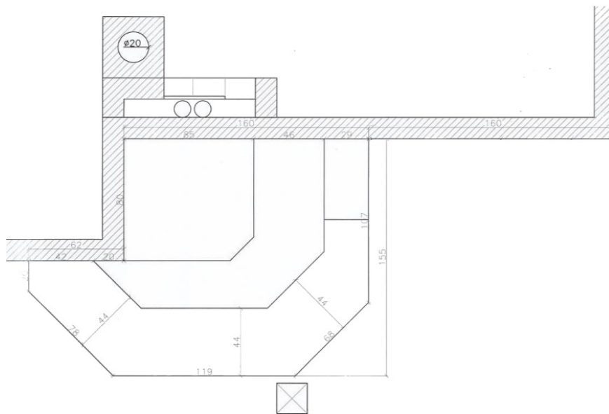
Slika 23: Tloris peči in prostorske situacije. (Gradbena dokumentacija)
